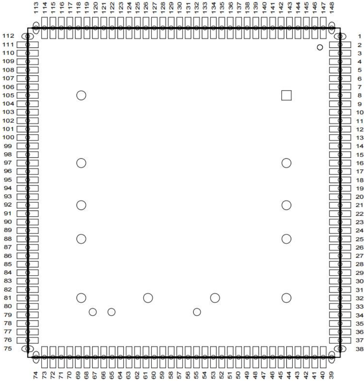
图 3-2 模块反面图
