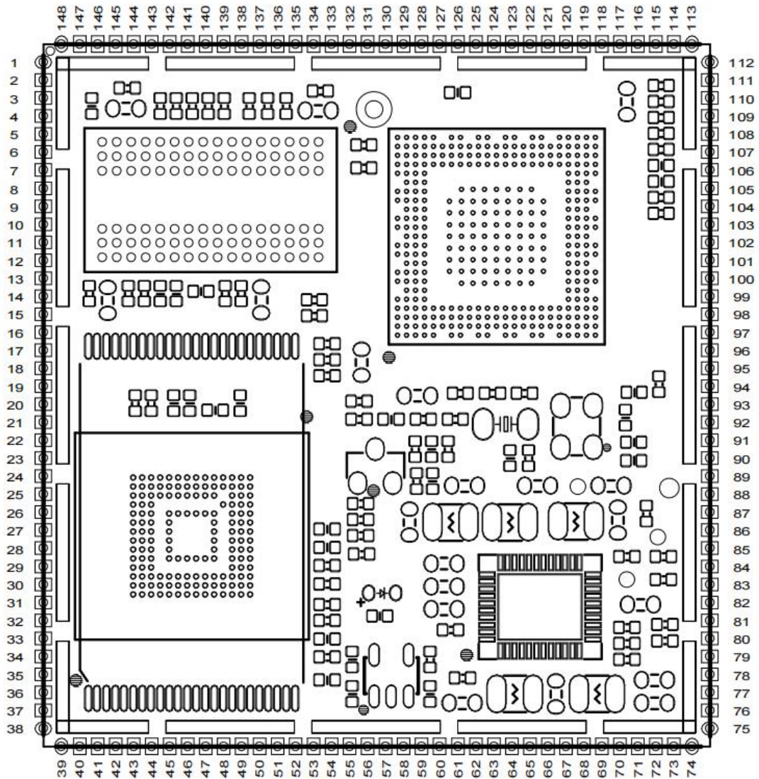
图 3-1 模块正面图
